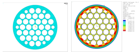
図 1: 入り口電極。左)モデリング図、右)2000℃一様分布時の変形量分布。電極大きさはφ12.7 mm である。
